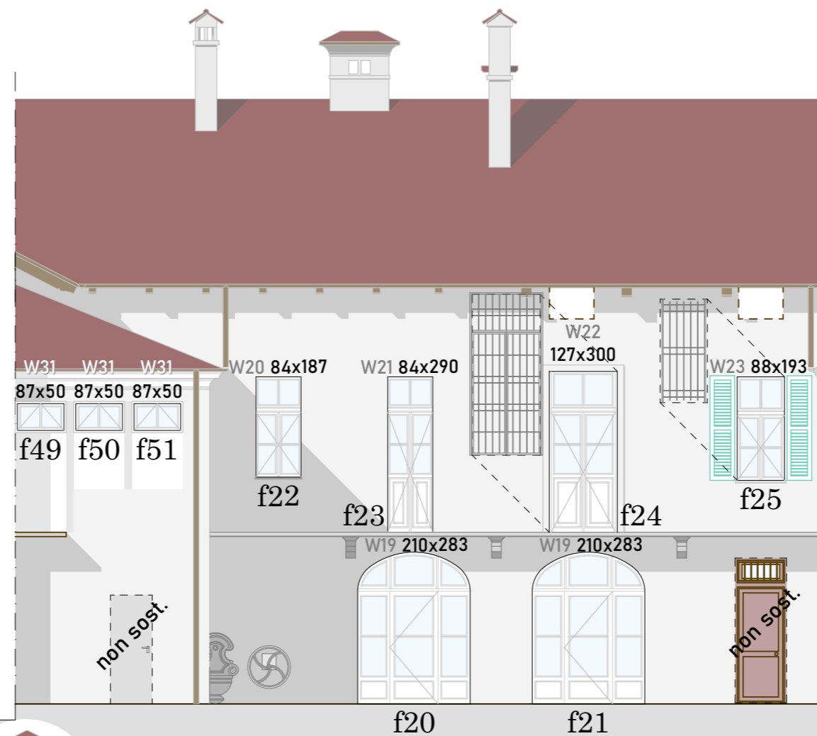
PROSPETTO NORD Corte ovest
