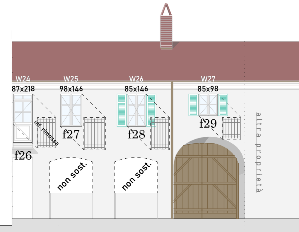
PROSPETTO EST Corte ovest
