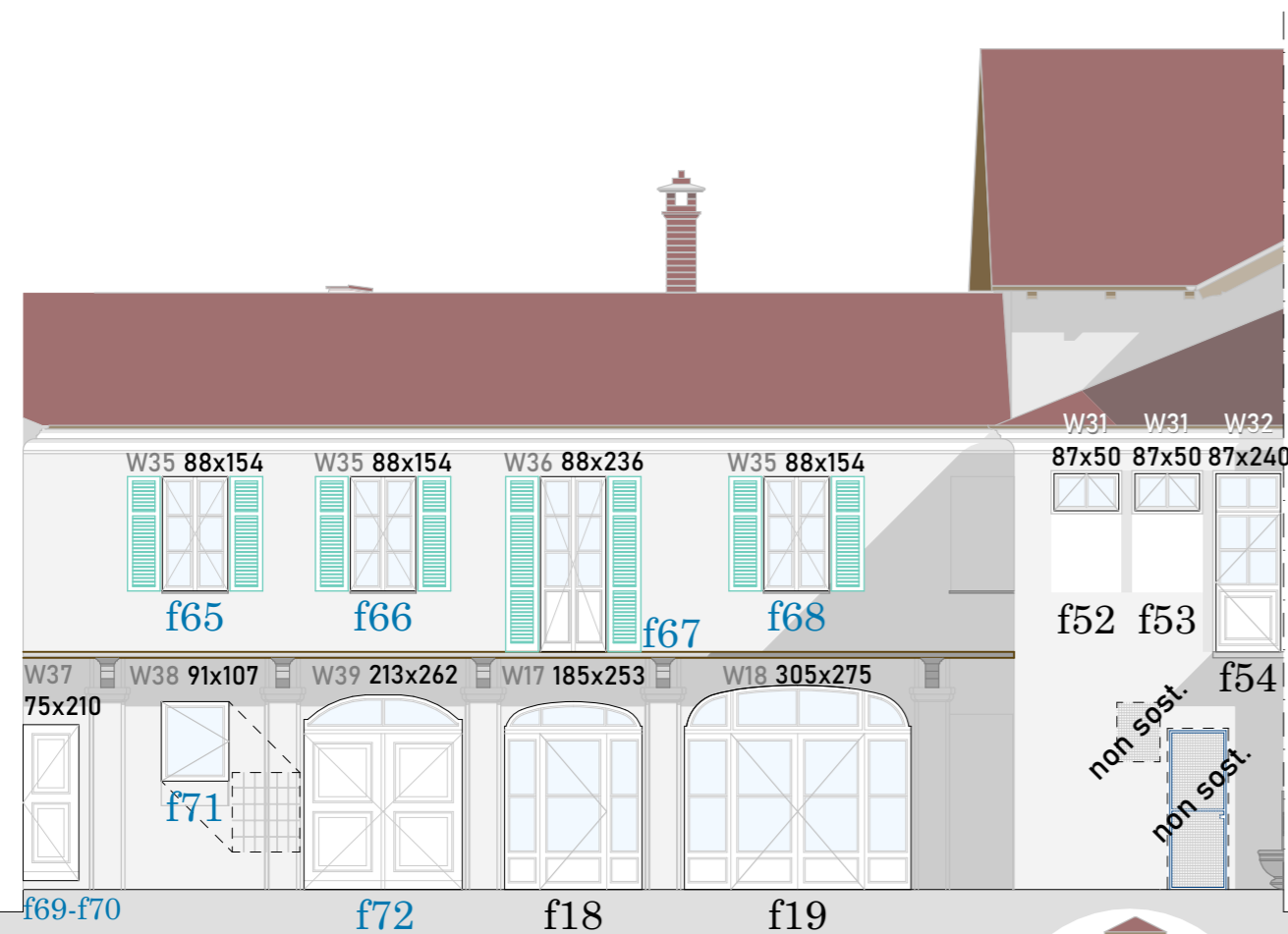
PROSPETTO OVEST Corte ovest
