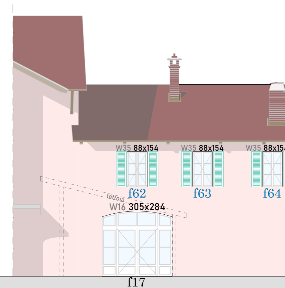
PROSPETTO EST Corte est
