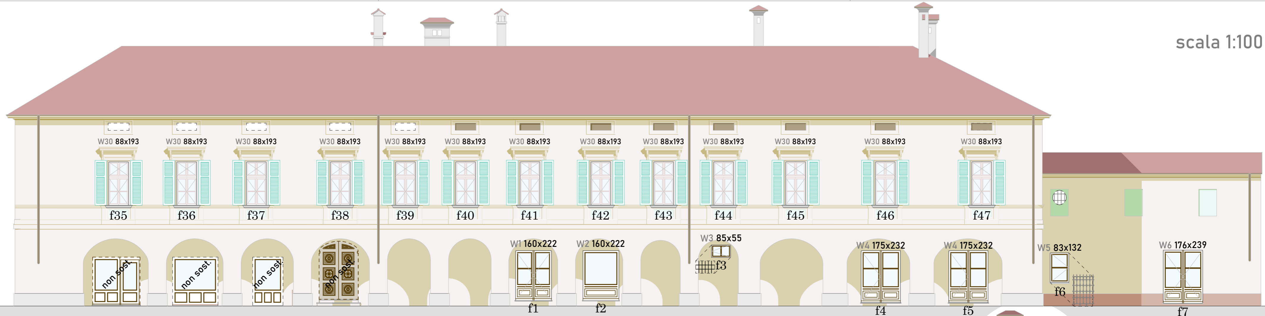
PROSPETTO SUD Via Umberto I
