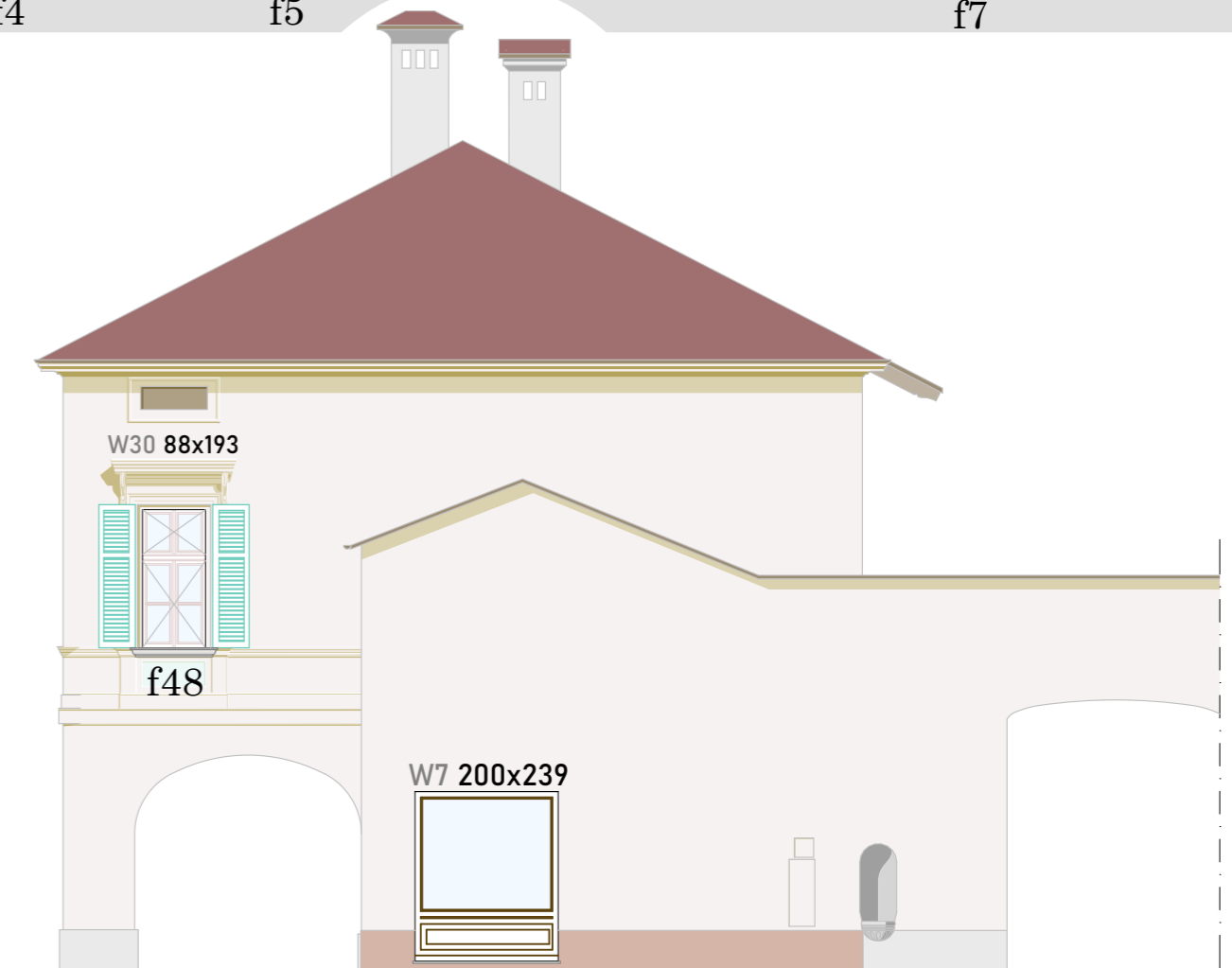
PROSPETTO EST Vicolo Arnaldi di Balme
